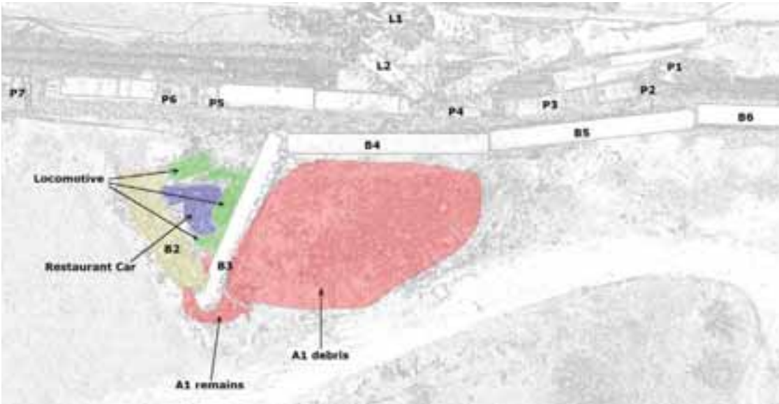
Σχήμα 12. Ο χώρος του δυστυχήματος. Οι θέσεις των μηχανών L1 και L2 της εμπορικής αμαξοστοιχίας και τα βαγόνια της P1 - P7. Το «μπάζωμα» και οι γερανοί έγιναν αριστερά του B3 (3ο βαγόνι της επιβατικής). Ο χώρος A1 debris, δηλ. συντρίμια του βαγονιού A1 της πρώτης θέσης, έμεινε απείραχτος.
