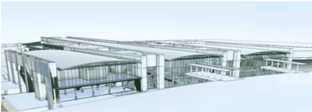
Για το αεροδρόμιο Λάρνακας οι εργασίες προνοούν επέκταση του τερματικού κτηρίου, την κατασκευή νέων πυλών επιβίβασης/αποβίβασης επιβατών με τη δημιουργία μιας νέας πτέρυγας που θα ενώνεται με το κυρίως κτήριο.
