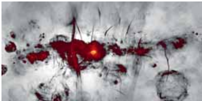
Η εικόνα, από το ραδιοτηλεσκόπιο MeerKAT, αποκαλύπτει μια καταιγίδα δραστηριοτήτων στην κεντρική περιοχή του γαλαξία μας.
