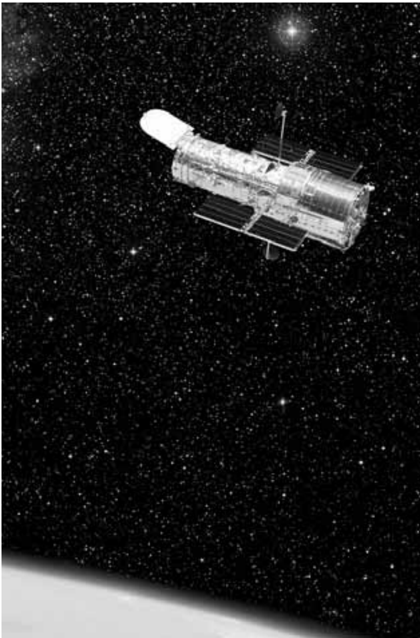
Το διαστημικό τηλεσκόπιο Χαμπλ βρίσκεται πάνω από την περιοχή της γήινης ατμόσφαιρας που παραμορφώνει τις αστρονομικές παρατηρήσεις, πολύ πάνω από τα σύννεφα της βροχής και τη φωτεινή ρύπανση και έτσι έχει ανεμπόδιστη θέα στο Σύμπαν.
