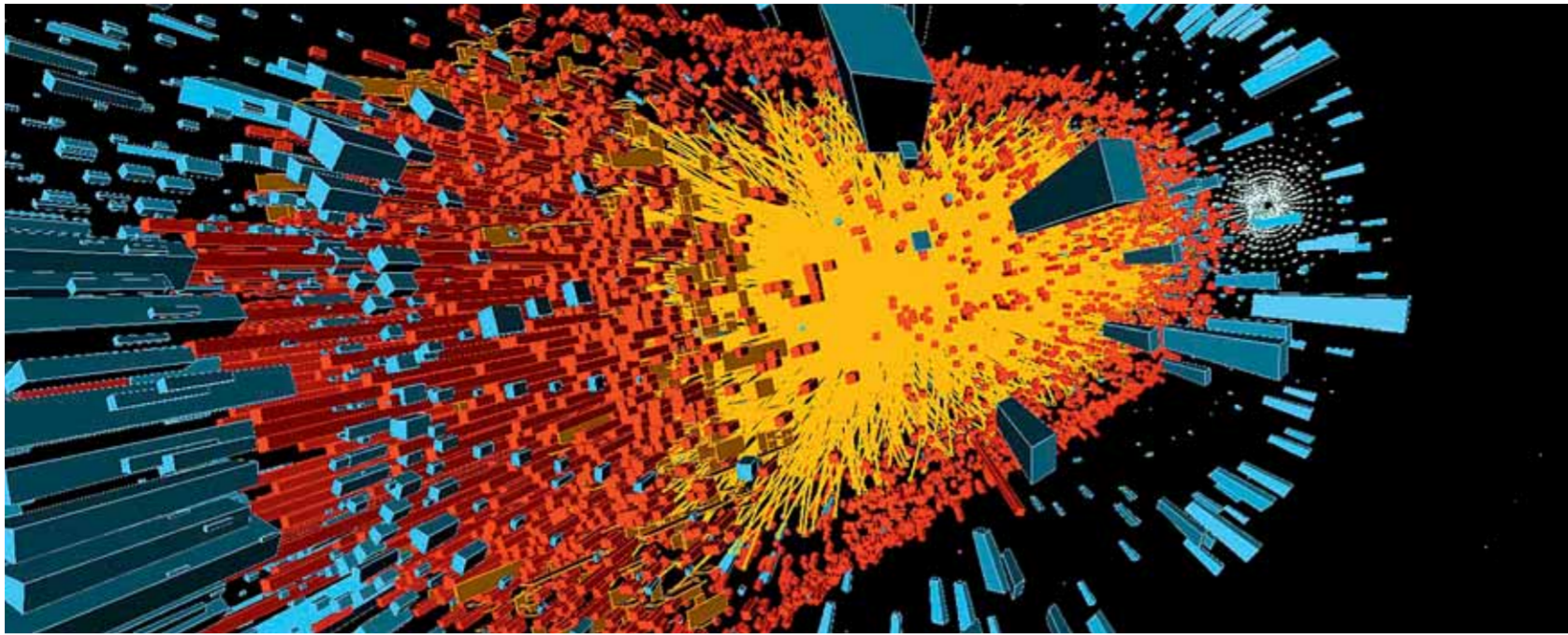
Το πείραμα της 7ης Νοεμβρίου πέτυχε και οι επιστήμονες του CERN μπόρεσαν μέσω συγκρούσε ιόντων μολύβδου να δημιουργήσουν μια «Μεγάλη Εκρηξη».
